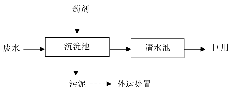
图4-1 本项目废水处理工艺流程图
